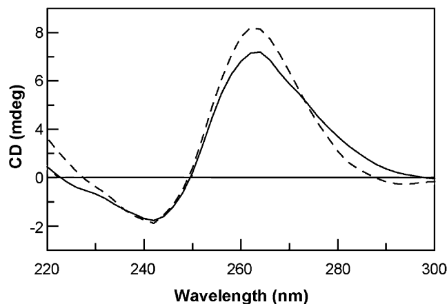
Figure 1. CD spectra of I (—) and II (---).
