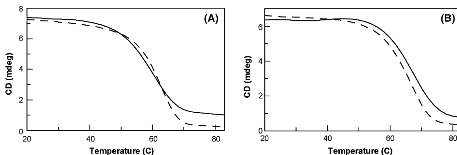
Figure 6. CD thermal denaturation profile of [d( A^{8Me} GGGT)] 4 ( I ) (—) and [d(AGGGT)] 4 (---) (A); [d( TA^{8Me} GGGT)] 4 ( II ) (—) and [d(TAGGGT)] 4 (---) (B).
